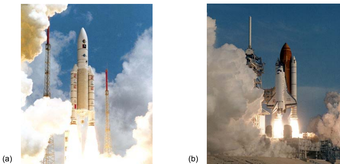
Figure 8. Propulsion de fusées à liquides cryogéniques (a) Ariane 5 (25 t H 2 , 130 t O 2 ) (b) Navette spatiale américaine (100 t H 2 , 600 t O 2 )
