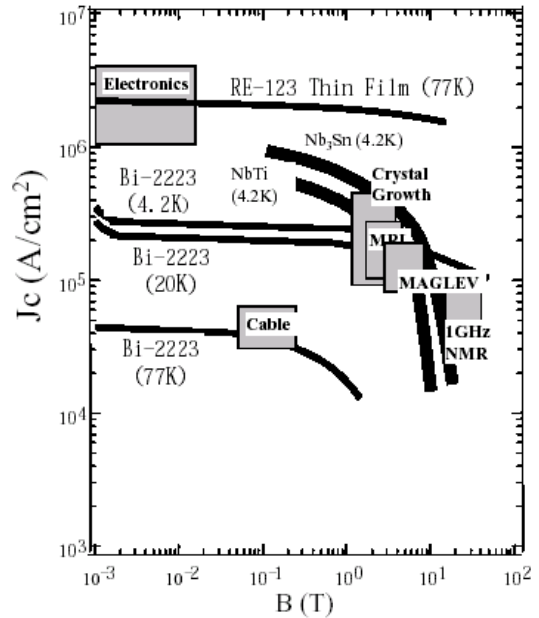
Figure 6. Performance des HTS industriels (BSCCO 2223) et champs d'application 7
