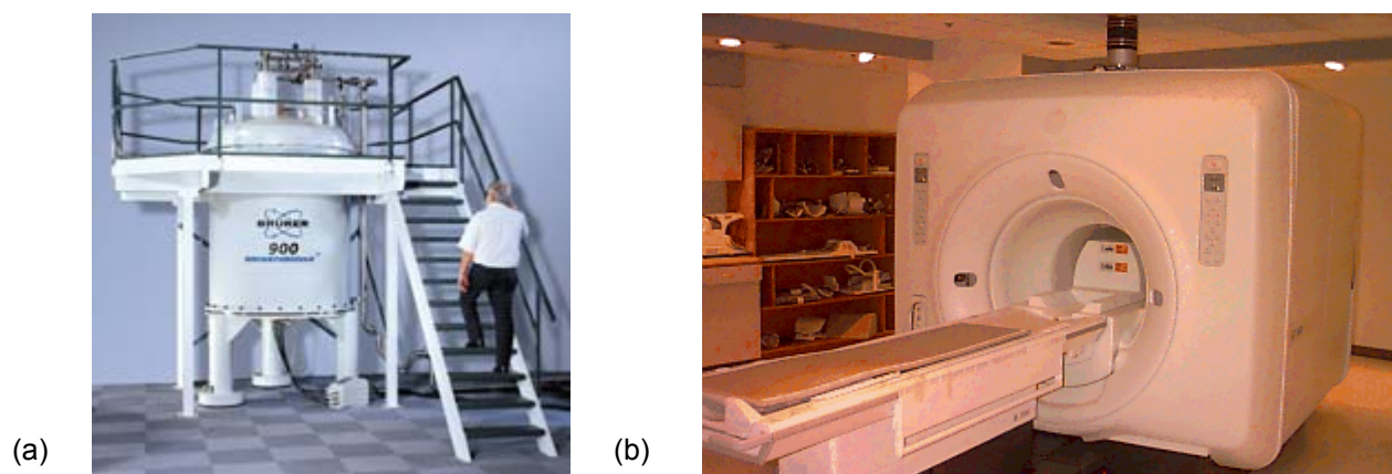
Figure 3. Aimants pour (a) RMN à 900 MHz, refroidi par de l'hélium superfluide, et (b) appareil utilisé pour la IRM du corps entier, refroidi par un bain d'hélium avec écran refroidi (Bruker)
