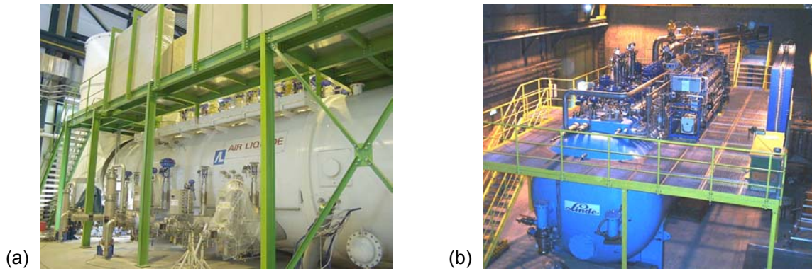
Figure 9. Installations cryogéniques à hélium de 18 kW à 4,5 K pour le LHC par (a) Air Liquide et (b) Linde
