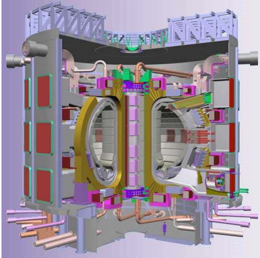
Figure 5. Le tokamak ITER, une machine de fusion par confinement magnétique en développement
