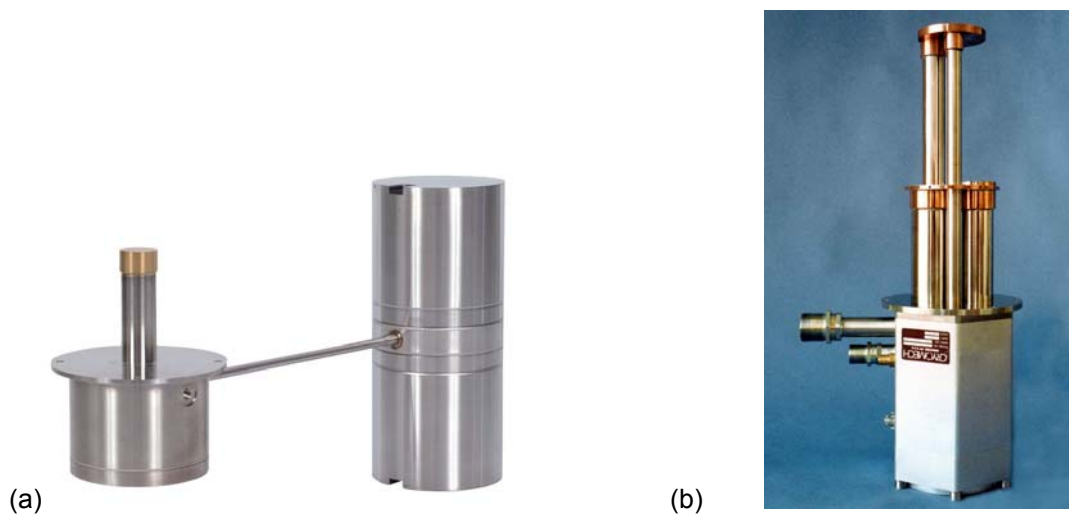
Figure 10. Refroidisseur Stirling linéaire monoétagé pour les applications spatiales avec un temps moyen entre défaillances de 20 000 heures (Thales) ; (b) Refroidisseur biétagé à tube pulsé fonctionnant à 4 K (Cryomech)
